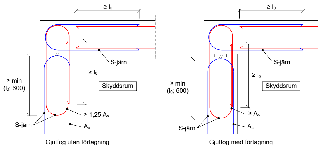
Figur 6:43b. Schematisk illustration för utförande av gjutfog när mötande armeringsslingor placeras omedelbart utanför hörnområdet. Mått i mm.
