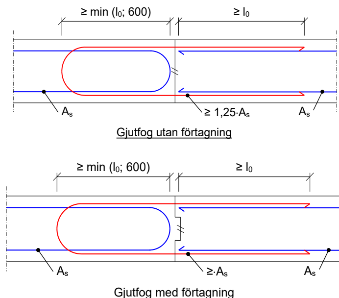
Figur 6:43c. Utförande av gjutfog när mötande armeringsslingor placeras i fält Mått i mm.
