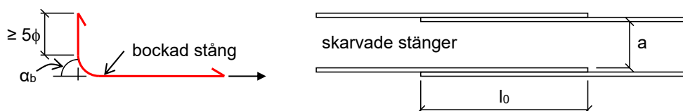
Figur 6:41a. Definition av bockningsvinkel \alpha_b och fritt avstånd a mellan stänger.
