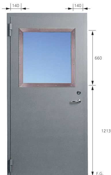
Glasöppning 24
